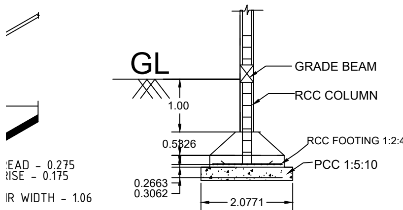
SECTION ON - BB (N.T.S)
