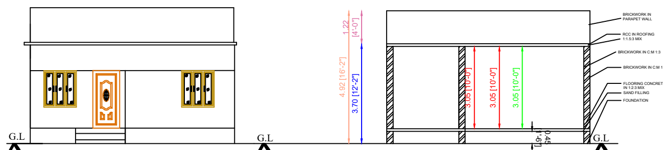
ELEVATION
