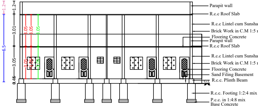
SECTION A-B
