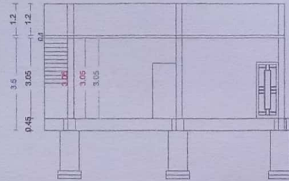
SECTION A-B
