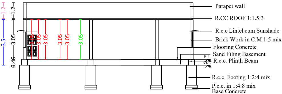
SECTION A-B
