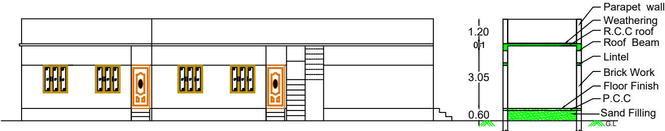
ELEVATION
