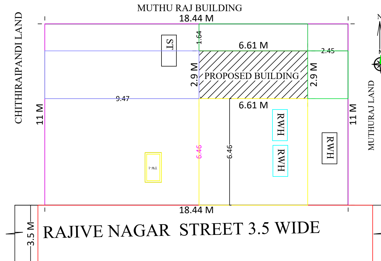
SITE PLAN 1:100 SCALE
