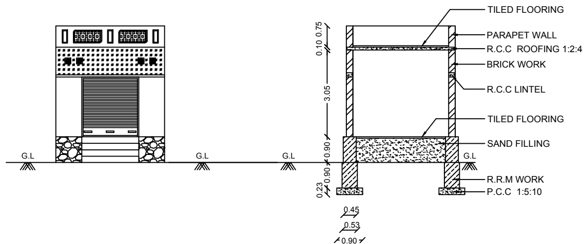
ELEVATION
