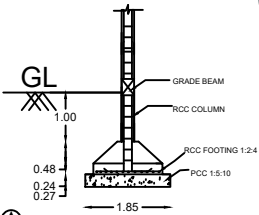
SECTION ON - BB (N.T.S.)
