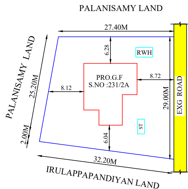
SITE PLAN (Scale 1:300)
