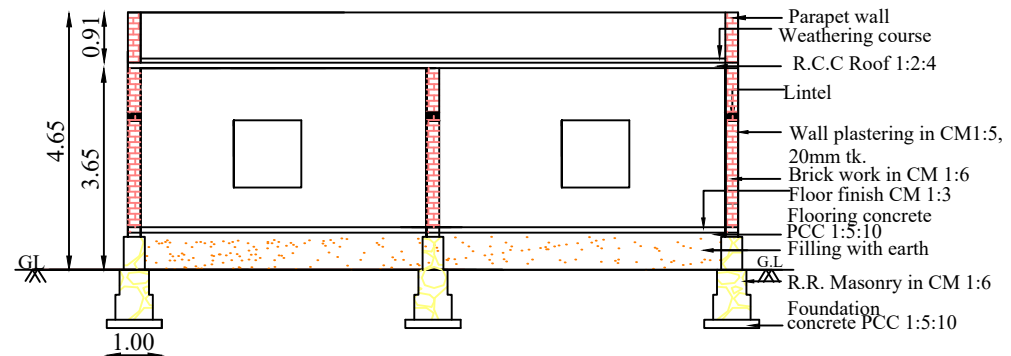
SECTION A-B
