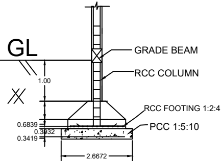
SECTION ON - BB (N.T.S)
