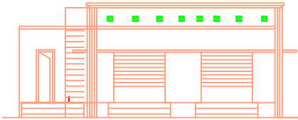
ELEVATION
