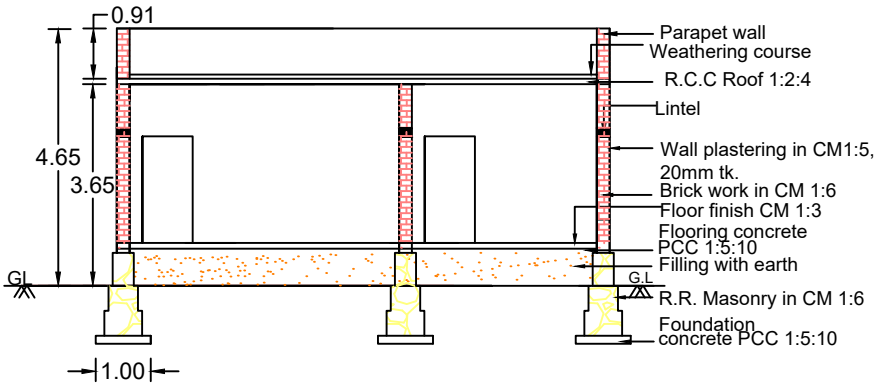
SECTION A-B
