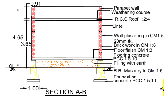
SECTION A-B
