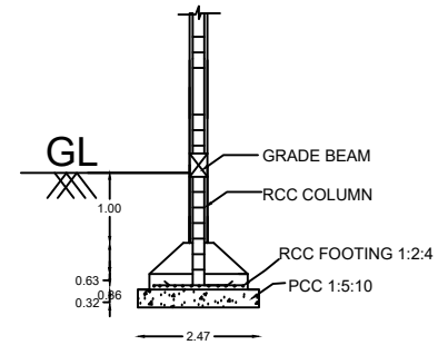
SECTION ON - BB (N.T.S)
