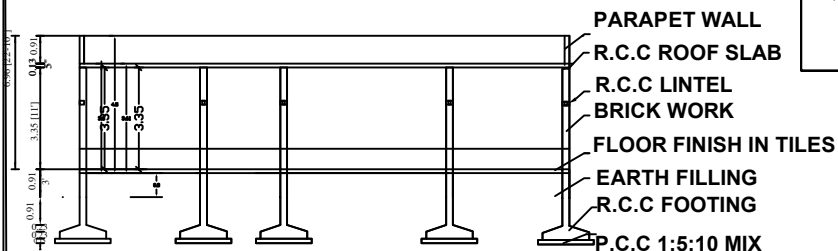
ELEVATION
