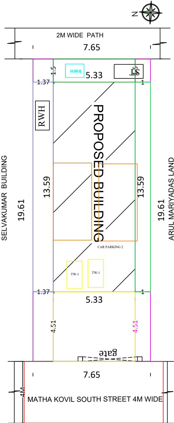
SITE PLAN 1:100 SCALE
