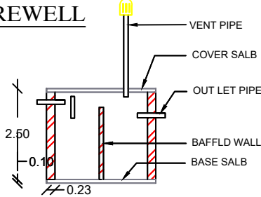
SECTION ON X - Y
