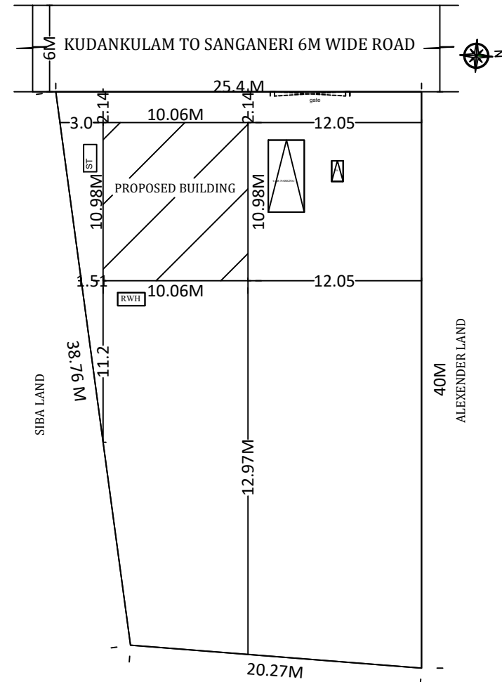
SITE PLAN 1:100 SCALE
