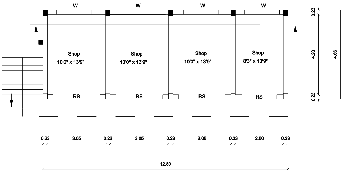
PRO.F.F PLAN
