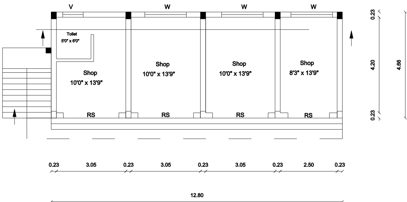
PRO. G.F PLAN
