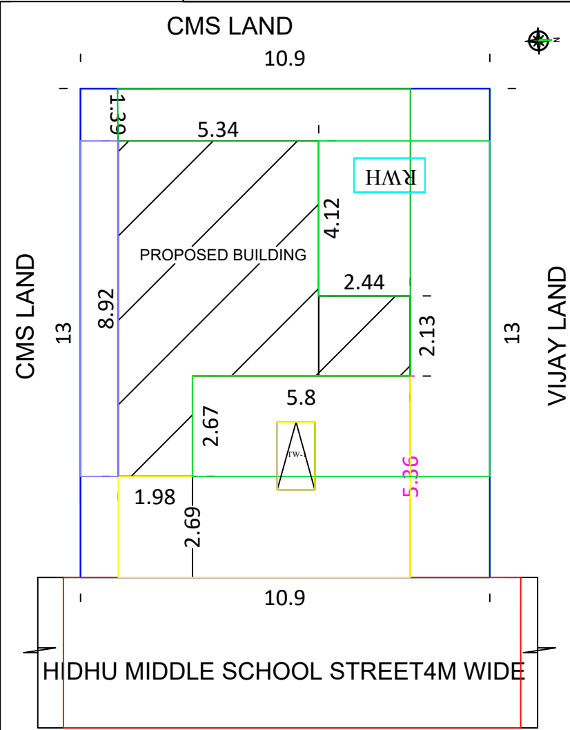
SITE PLAN 1:100 SCALE
