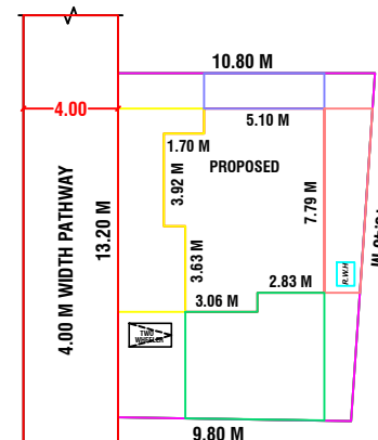
SITE PLAN SCALE 1:100
