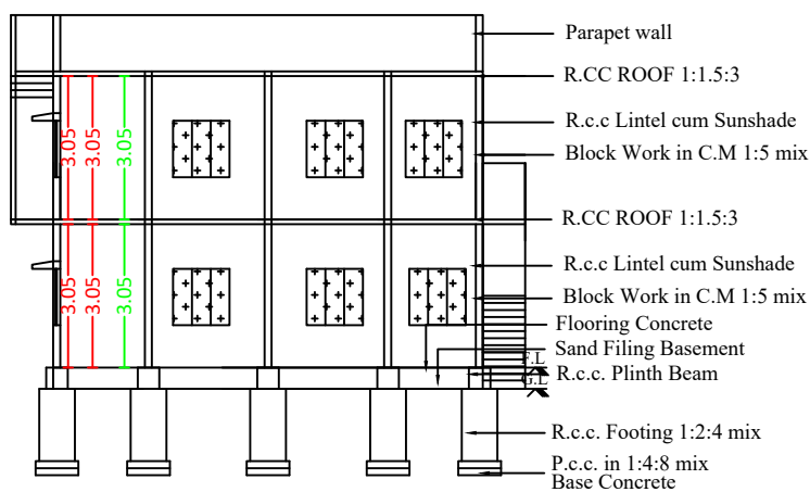
SECTION A-B
