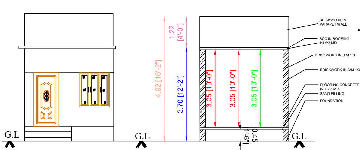
ELEVATION
