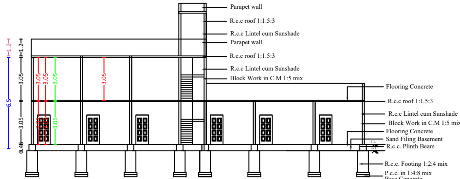
SECTION A-B
