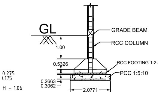
SECTION ON - BB (N.T.S.)
