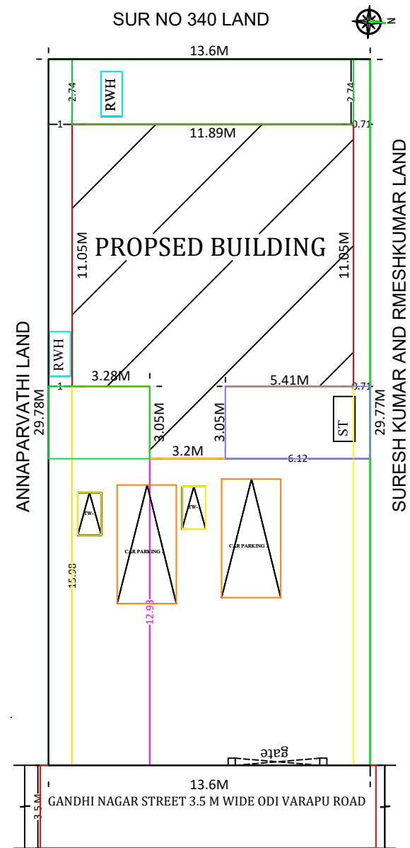
SITE PLAN 1:100 SCALE
