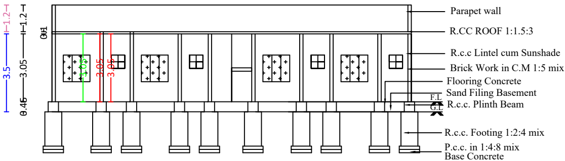
SECTION A-B
