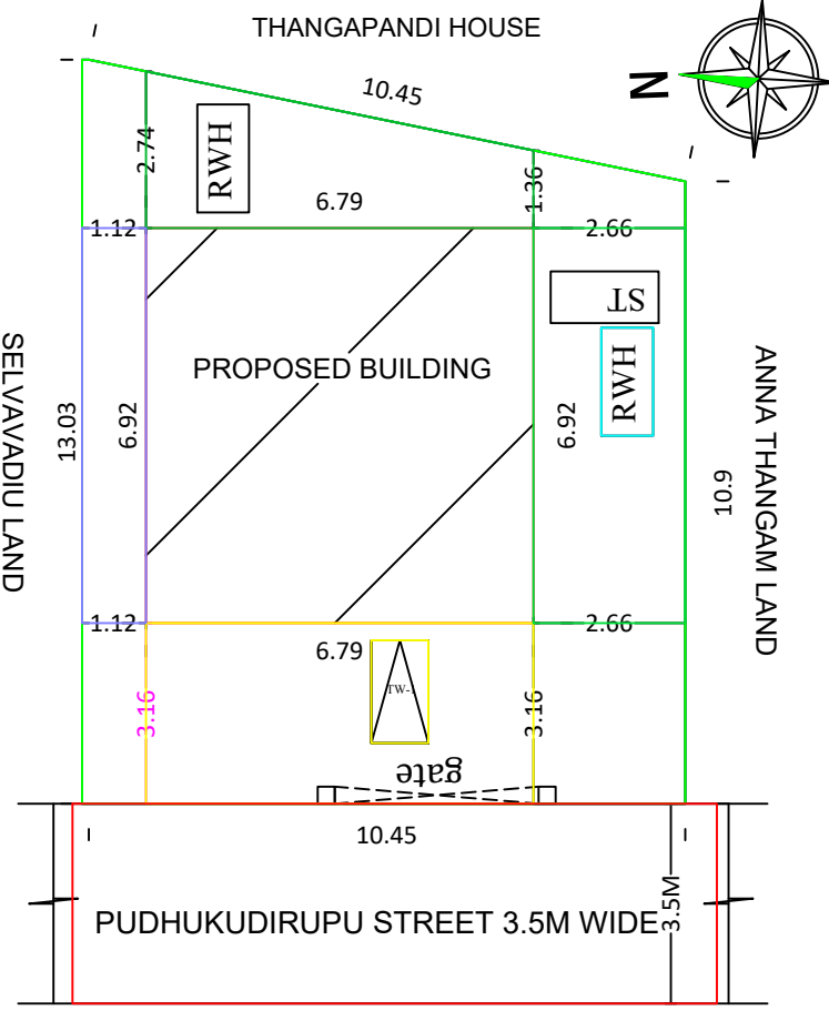
SITE PLAN 1:100 SCALE
