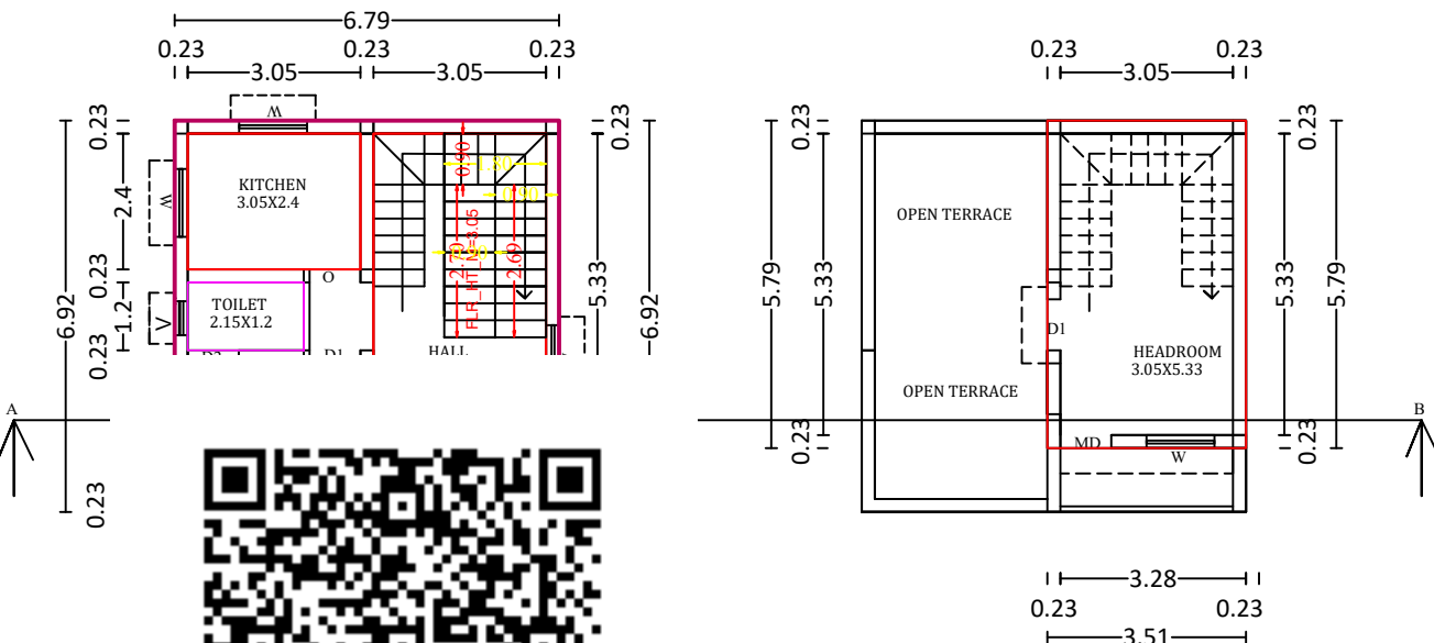
F.F PLAN
