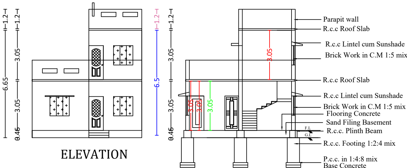
SECTION A-B
