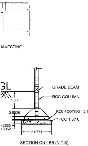
SECTION ON - BB (N.T.S)
