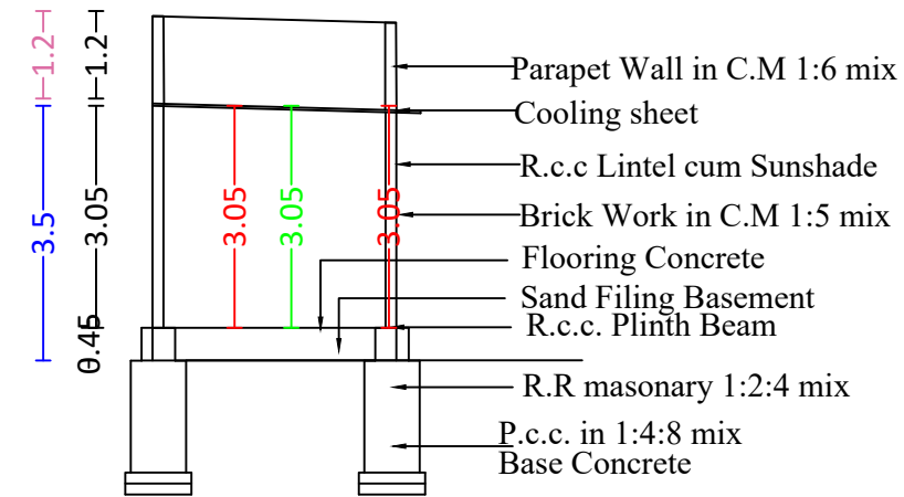
SECTION A-B
