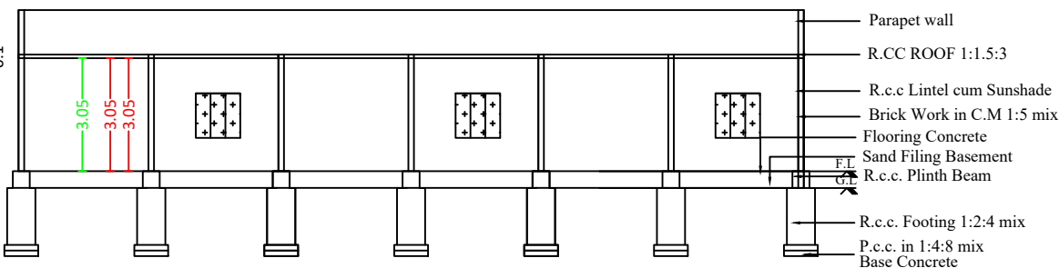
SECTION A-B
