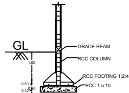
SECTION ON - BB (N.T.S)
