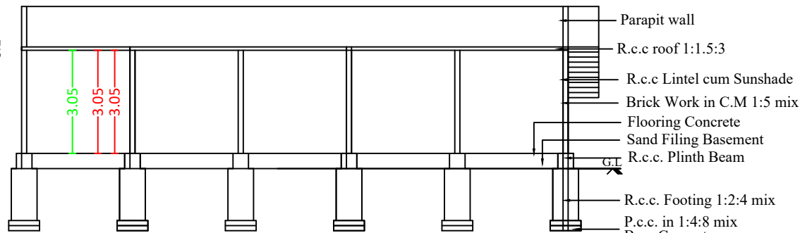
SECTION A-A
