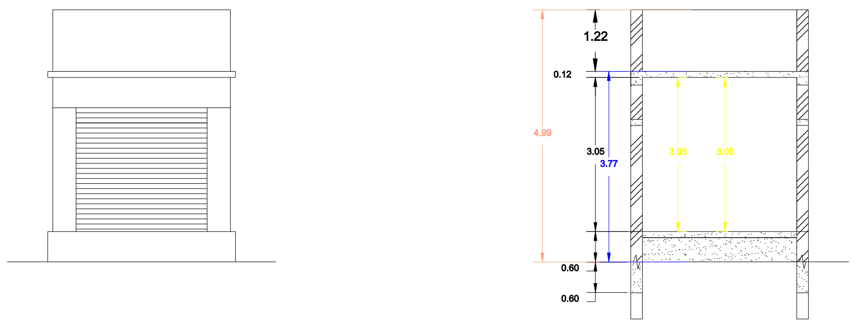
ELEVATION
