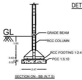
SECTION ON - BB (N.T.S)
