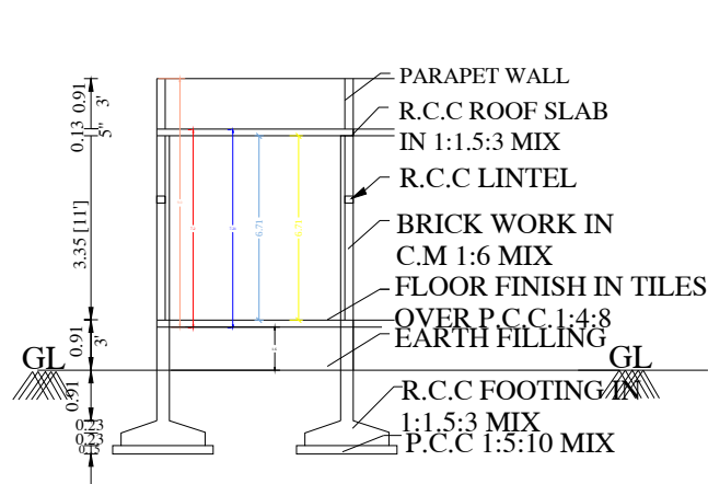
SECTION A-B
