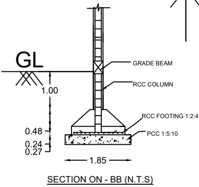
SECTION ON - BB (N.T.S)
