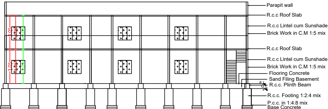
SECTION A-B
