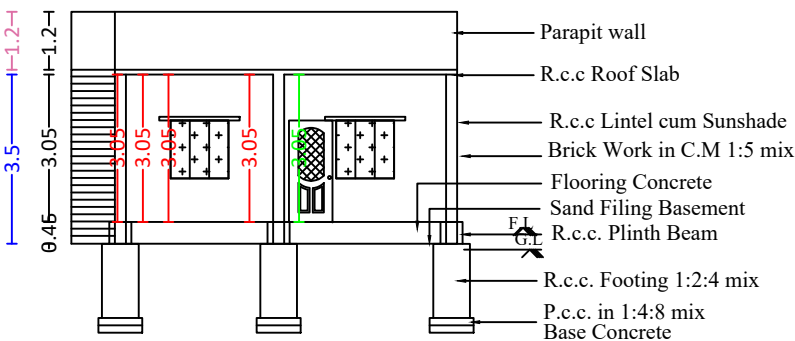
SECTION A-B
