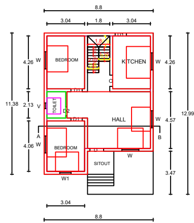
GRONUD FLOOR PLAN
