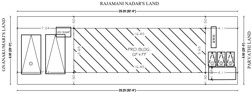
SITE PLAN 1:100
