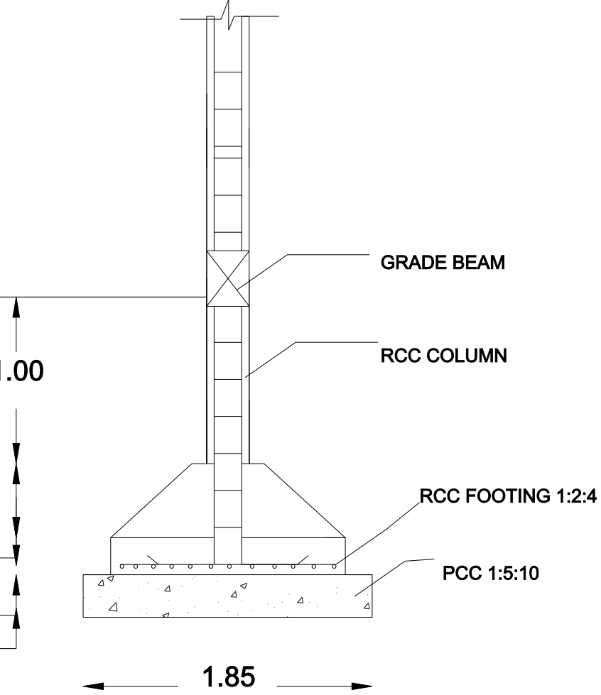
SECTION ON - BB (N.T.S)
