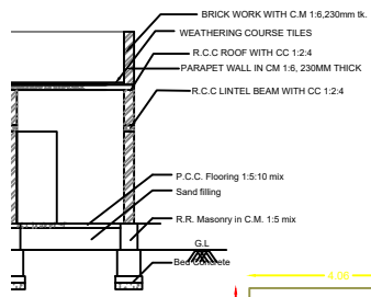
SECTION ON A-A (N.T.S)
