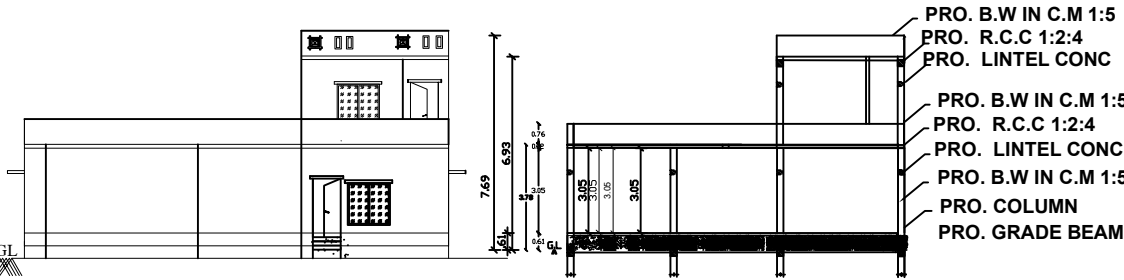
ELEVATION
