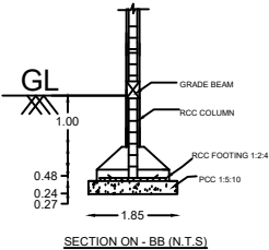
SECTION ON - BB (N.T.S.)
