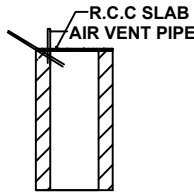
SOAK PIT
