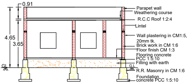
SECTION A-B
