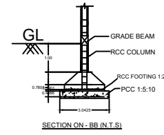
SECTION ON - BB (N.T.S)
