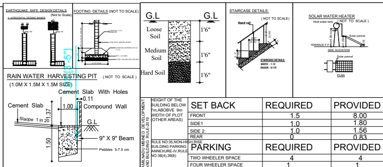
MURUGAN MANAI SITE PLAN(SCALE 1:100)
