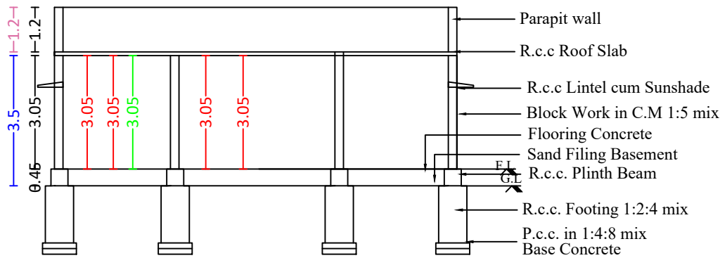
SECTION A-B
